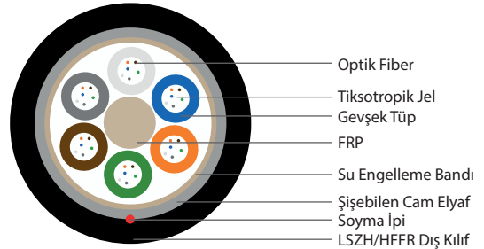
48 Fiber 6x8
