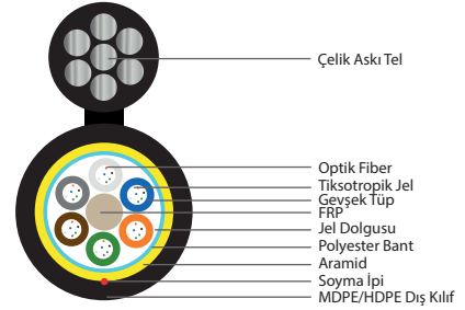
48 Fiber 6x8
